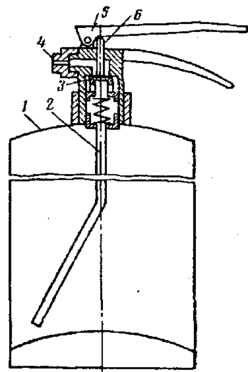
Рис. 4. ВВБ-3
