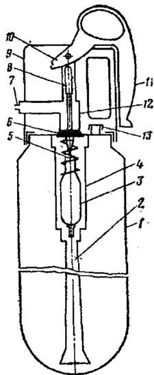
Рис. 6. ВП-1 "Момент-2П":
