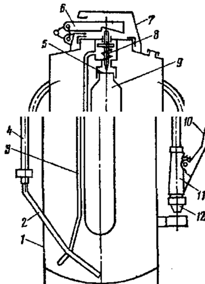
Рис. 5. ВП-10А:
