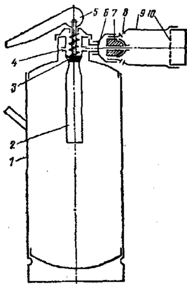
Рис. 2 ВХПП-10
